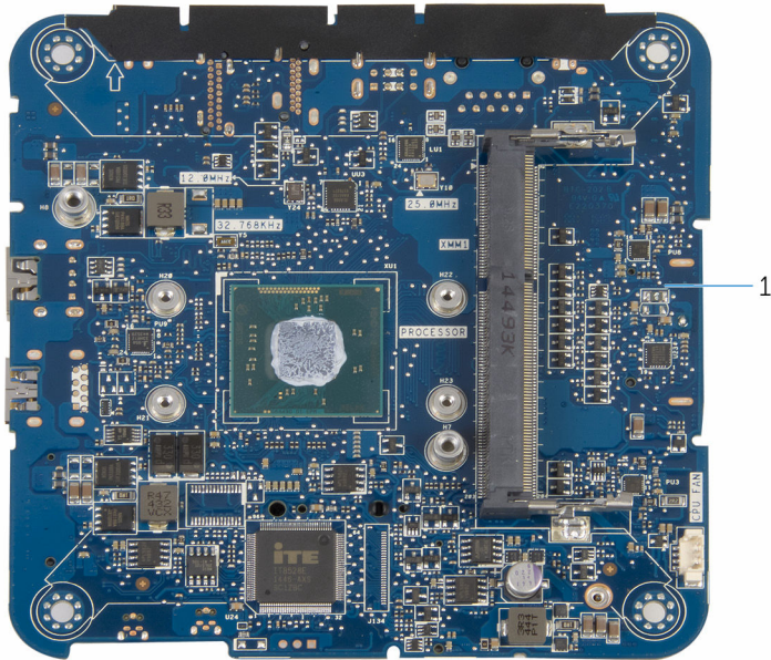
1 základní deska
